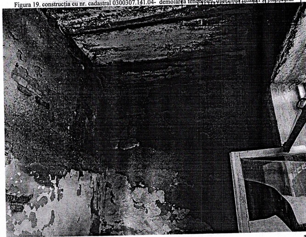
Figura 19. construcția cu nr. cadastral 0300307.141.04- demolarea tencuielei, umezirea zidăriei și planșoului
