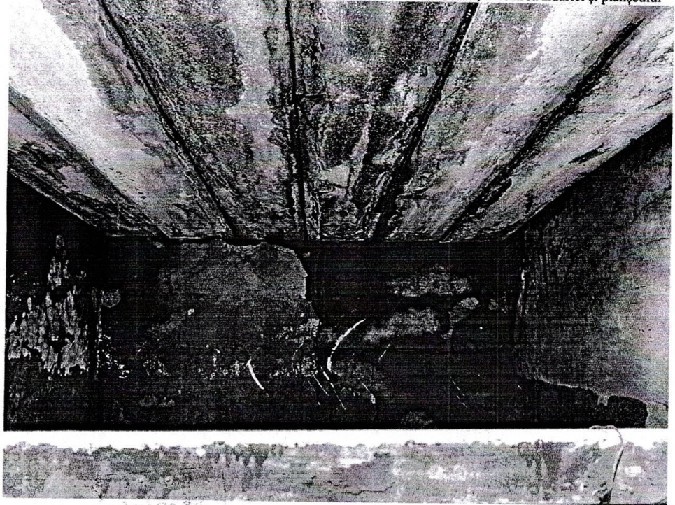
Figura 21. construcția cu nr. cadastral 0300307.141.04- coroziia grinzii din oțel
