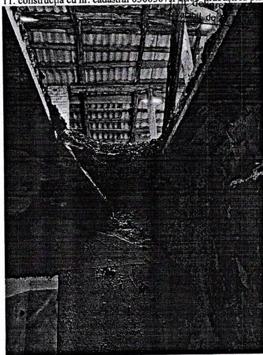
Figura 11. construcția cu nr. cadastral 0300307.141.03-prăbușirea planșeului
