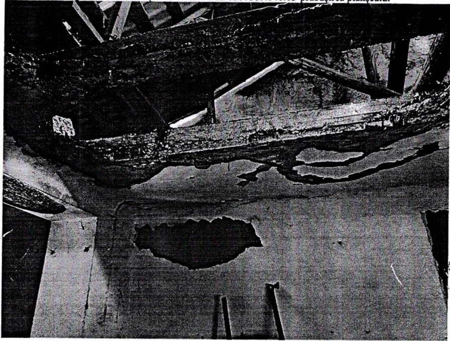
Figura 13. construcția cu nr. cadastral 0300307.141.03-prăbușirea planșului
